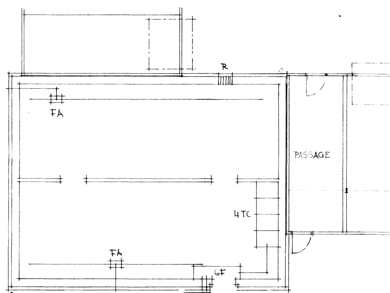
SKYDDSRUM FÖR 120 PLATSER
