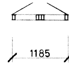
F4 ANTAL: 23 st 1. E1213 i princip glas: ytterbåge 8 mm maskinglas, innerbåge enl Sv. Riksb standard
