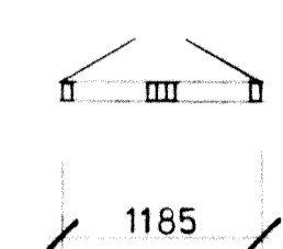
F 4 ANTAL: 23 st 1. E1213 i princip glas: ytterbåge 8 mm maskinglas, innerbåge enl Sv. Riksb standard
