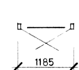
FD 3 ANTAL: 1 h 1. DB15F i princip mått enl figur glas: ytterbåge 4 mm maskinglas, innerbåge 2 x 4 mm maskinglas med 12 mm luftspält
