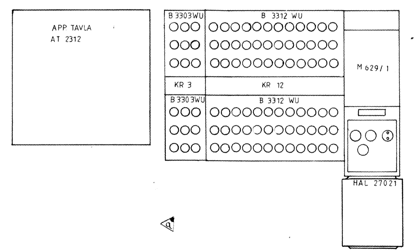
HUVUDCENTRAL I HUS K1
