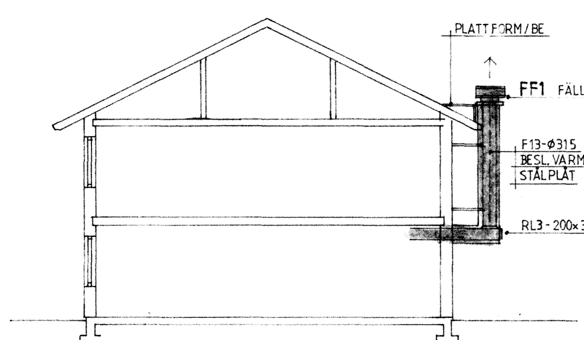
SEKTION A SKALA 1:100
