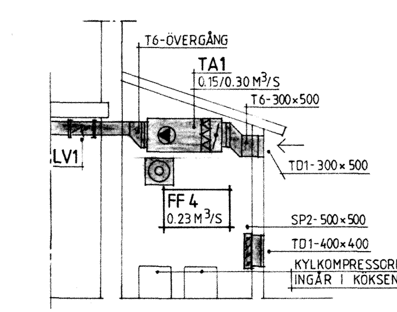
SEKTION B SKALA 1:100
